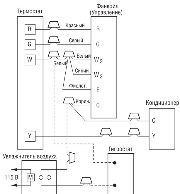
Рис. 22— монтажная схема подключения увлажнителя воздуха к фанкойлу с электрическим нагревателем
