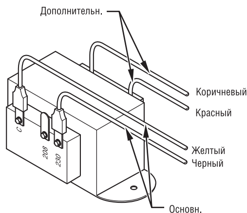
Рис. 14—Подключение трансформатора
